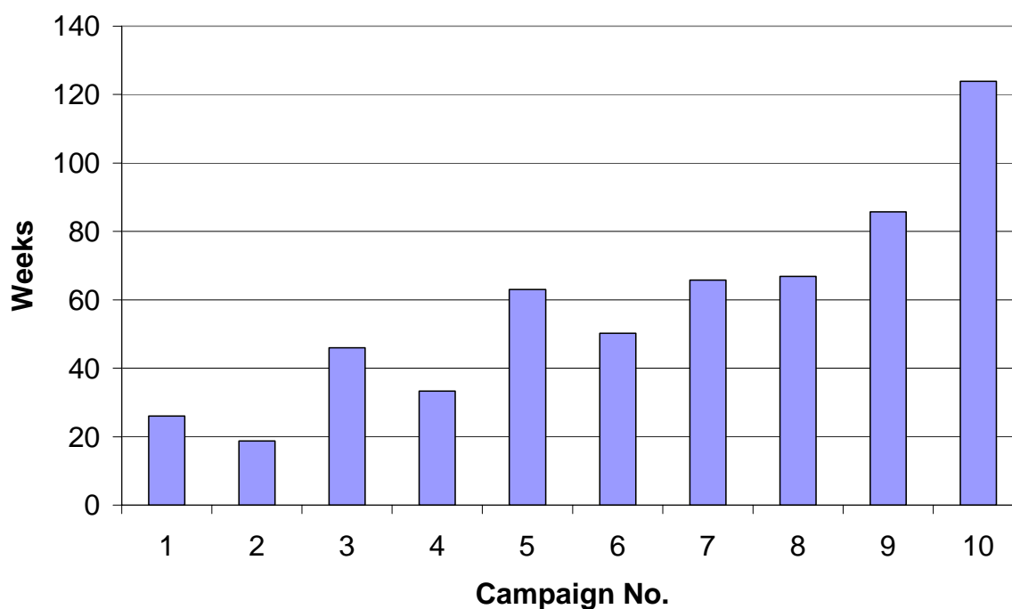
Figura 6 – Historial de duración de la campaña ISASMELT™ en Phelps Dodge Miami
