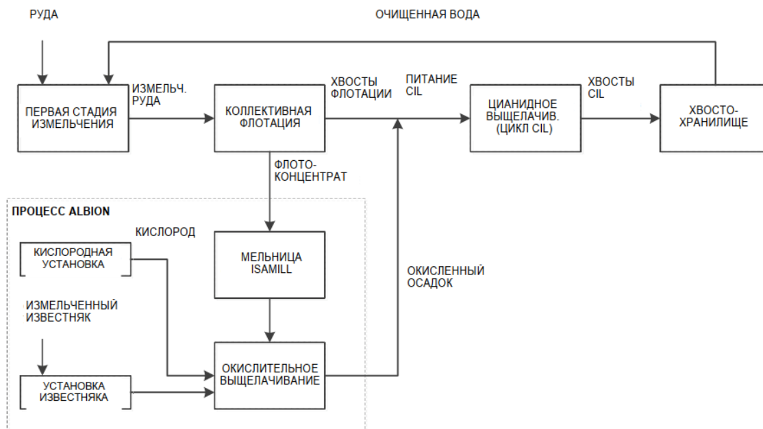
Рисунок 1 – Общая технологическая схема проекта ГПМ Голд
